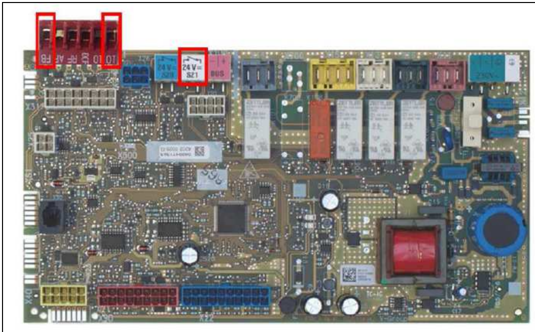
Szabályozó panel megjelölt EVU bemenettel (S21)
