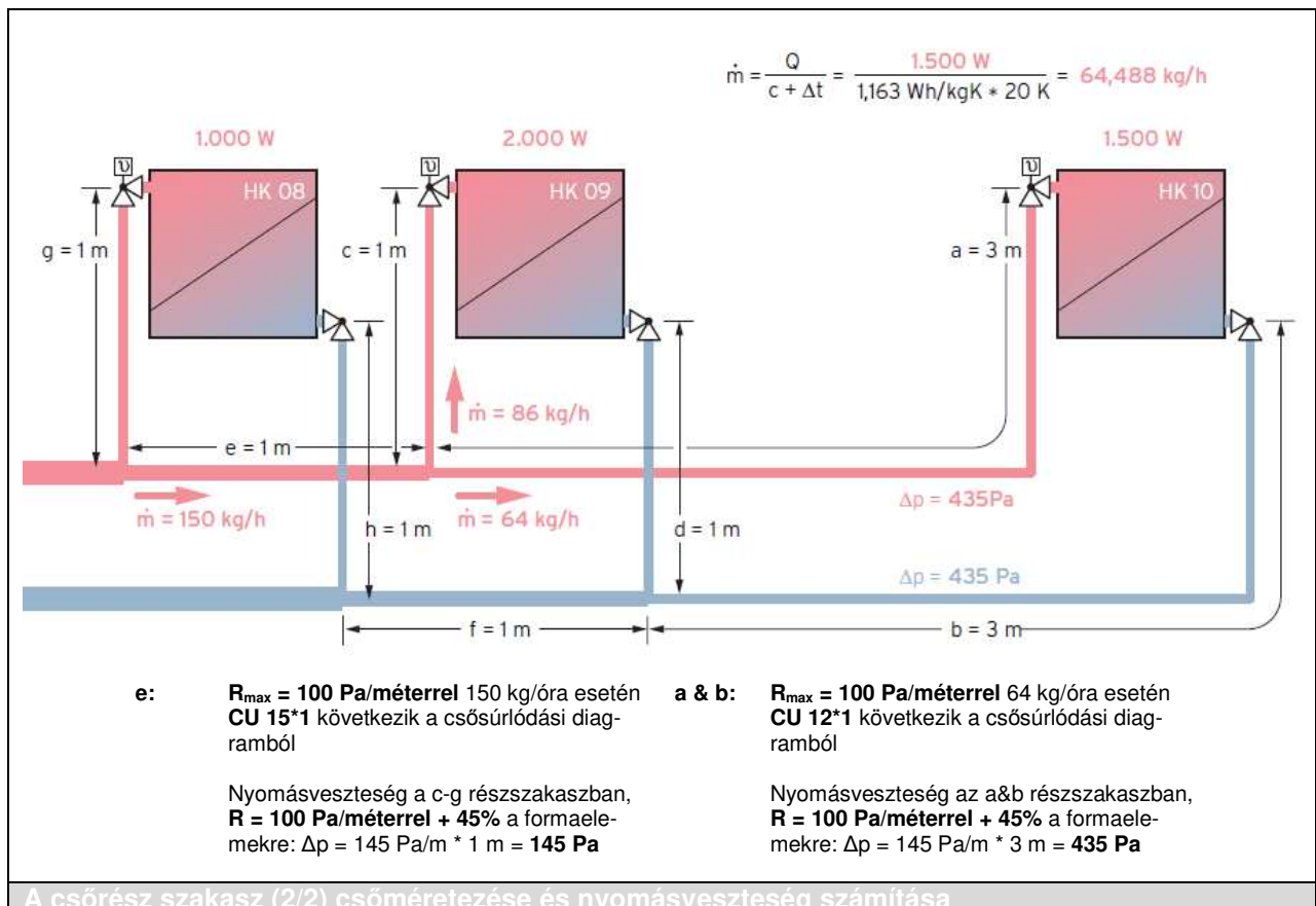
A cső rész szakasz (2/2) csőméretezése és nyomásvesztés számítása
