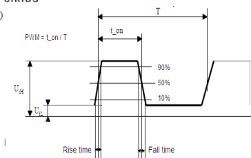
Figure Ábra 11. PWM hullám forma
