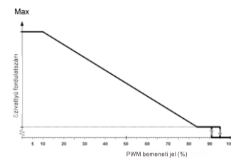
Ábra 13 PWM bemenet P1 (fűtés)
