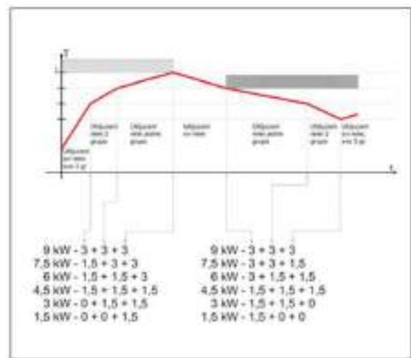
10. kép: Melegítő bekapcsolása és kikapcsolása
