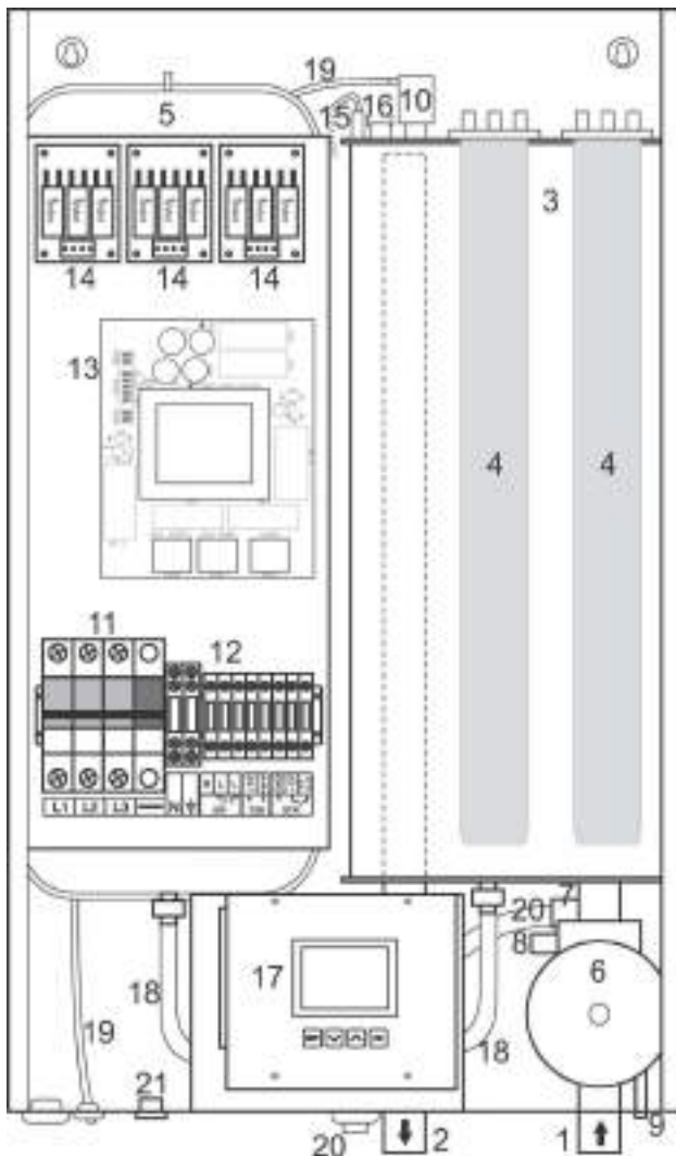
1. kép: Kazán részei
