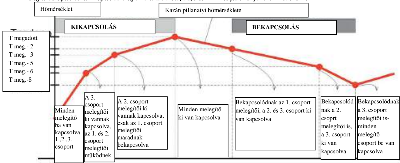
A melegítő bekapcsolási és kikapcsolási diagramja és táblázata, a 6, 9 és 12 kW teljesítményű kazán modellekhez
