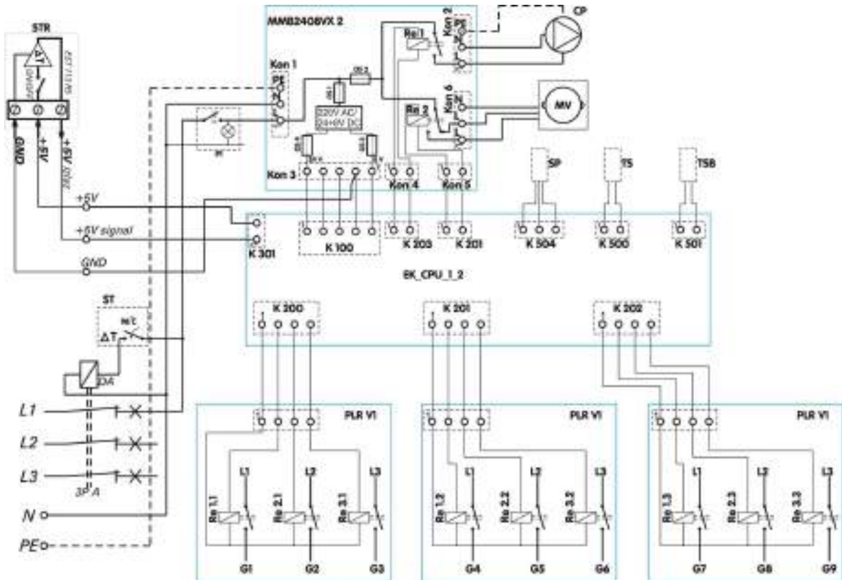
2.tábl: Compac ePlus EU összekapcsolási története és csatlakozási sémája
