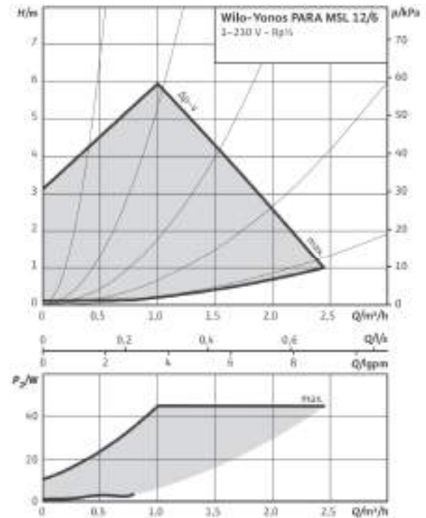
\Delta p-v (szivattyú váltakozó beállítása)
